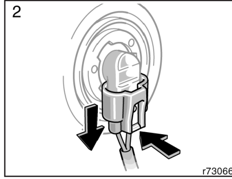
2. Kilit diline bastırarak soketi çıkarınız.
