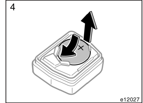
4. Pili şekilde gösterildiği gibi oynatınız. Kilidi çözülecek ve çıkarılabilecektir.
